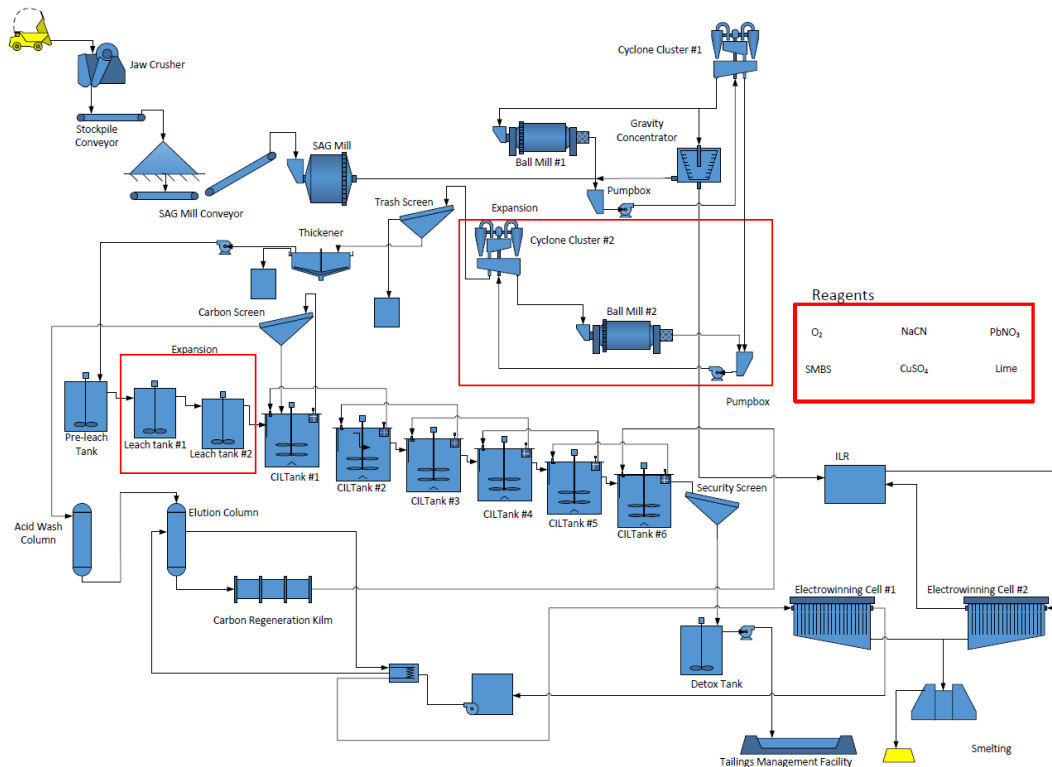
Figure 2: Schéma de traitement
