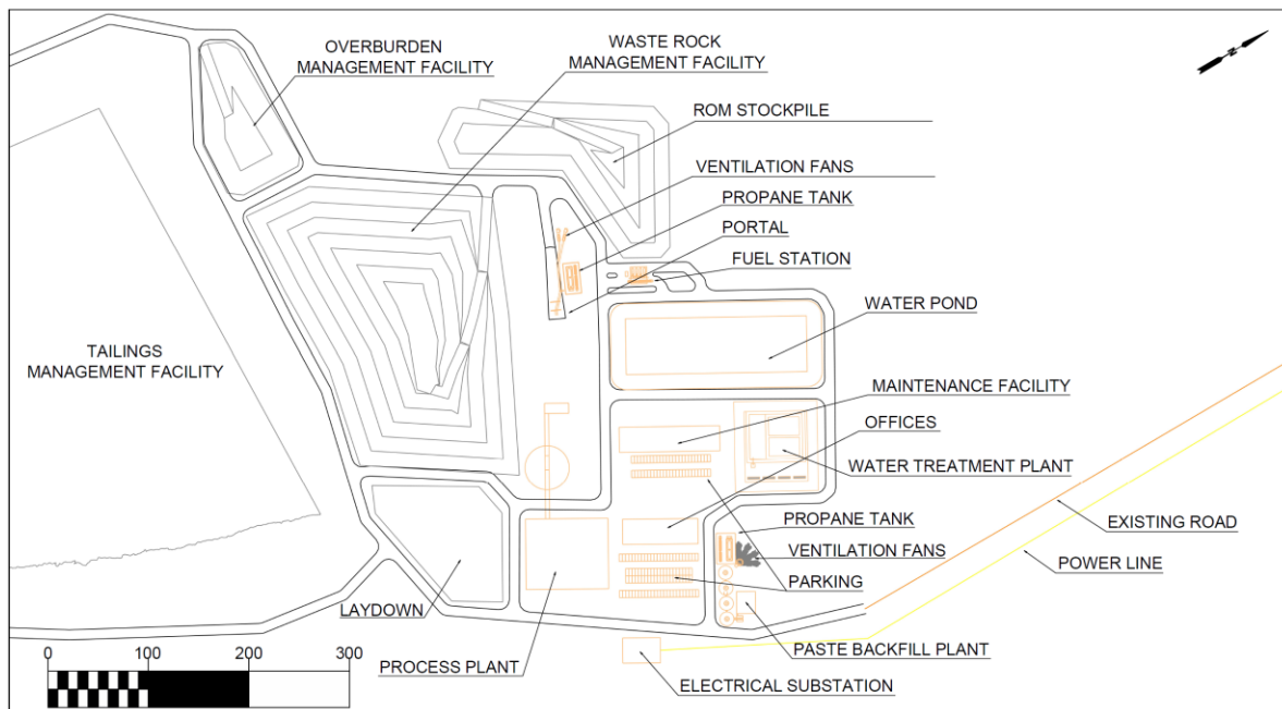
Figure 4: Infrastructures de la plateforme industrielle principale
